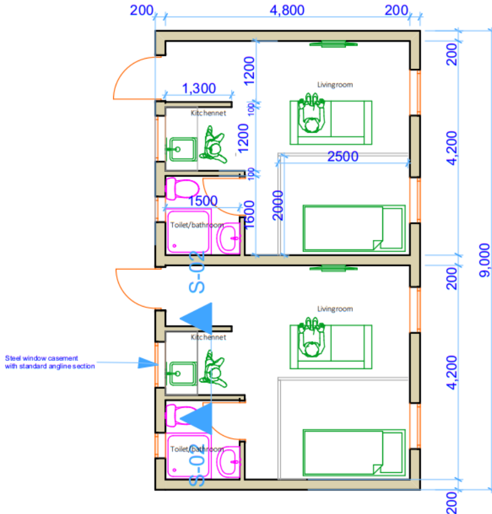
Bedsitter Type B
